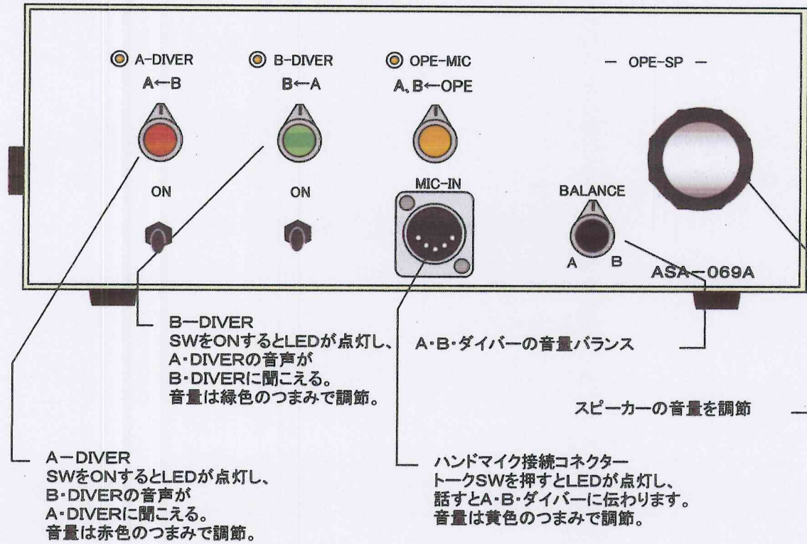
前パネル図
