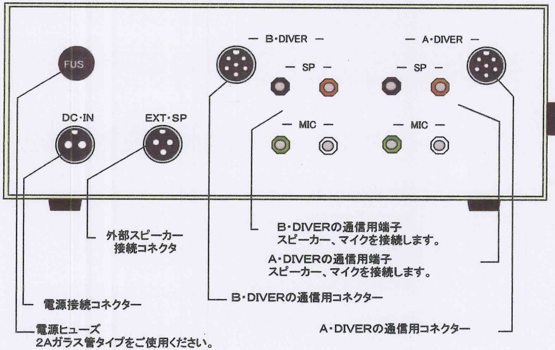
後パネル図
